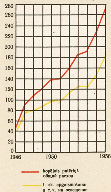
KOMUNALĀS SAIMNĒCĪBAS PĀTERĒTĀ ELEKTROENERĢIJA (milj. kWh) ПОТРЕБЛЕНО ЭЛЕКТРОЭНЕРГИИ КОММУНАЛЬНЫМ ХОЗЯЙСТВОМ (млн. квт-ч)
