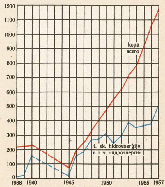
ELEKTROENERĢIJAS RAZOSANA (milj. kWh) ПРОИЗВОДСТВО ЭЛЕКТРОЭНЕРГИИ (млн. квт-ч)
