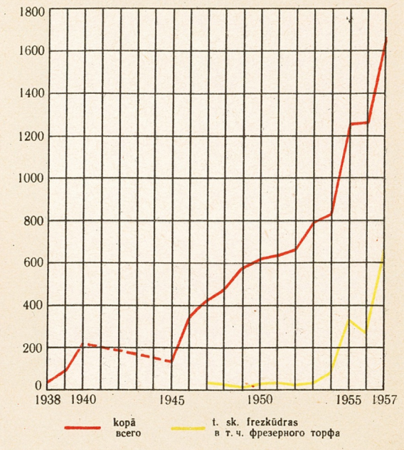
KURINĀMĀS KŪDRAS IEGUVE (tūkst. t) ДОБЫЧА ТОПЛИВНОГО ТОРФА (тыс. т)
